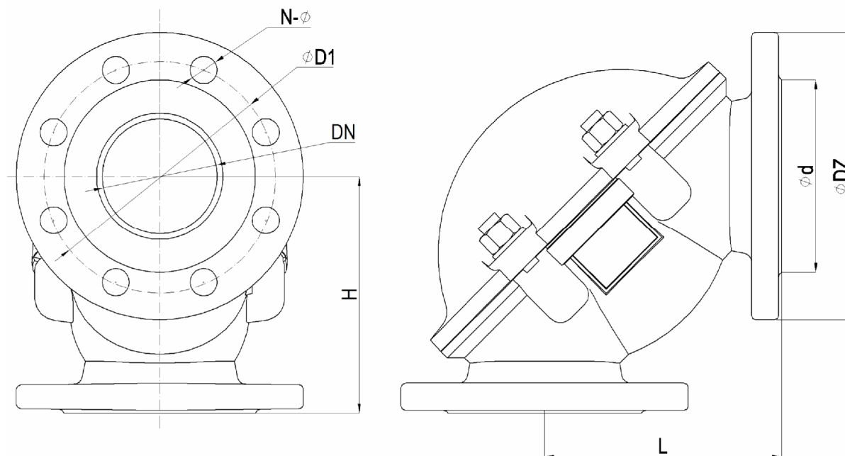
Рис. Обратный клапан в форме колена SZUSTER system тип TSK 02.
