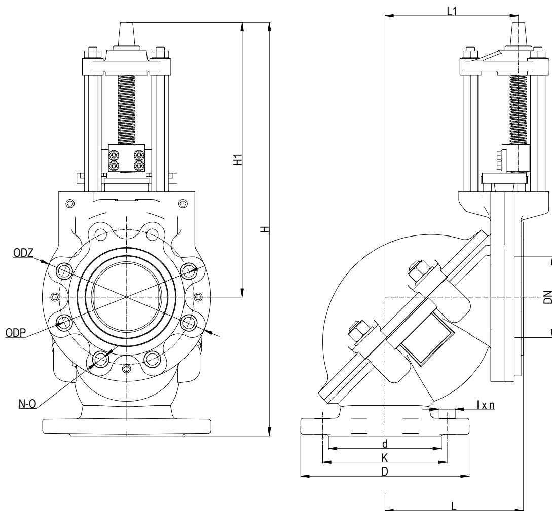
Рис. Коленчатый возвратный клапан Шустер (SZUSTER) система тип TSK COMBI 02.
