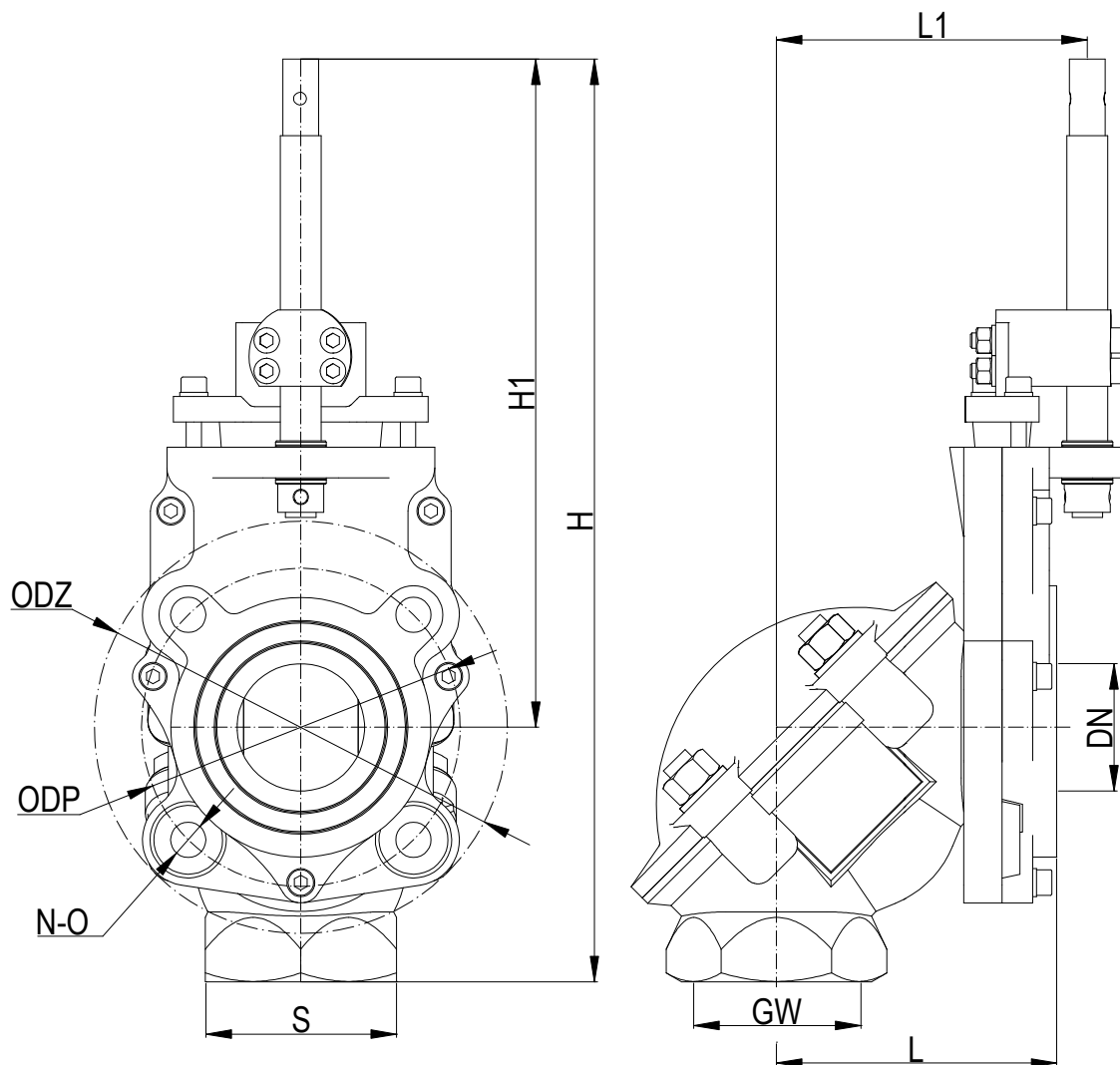
Рис. Коленчатый возвратный клапан Шустер (SZUSTER) система тип TSK COMBI 01.
