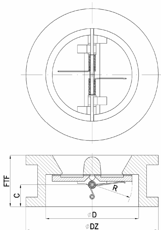
Рис. Обратный клапан тип ТКС.
