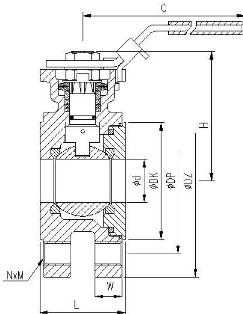
Фот. Шаровой клапан тип ZKM.
