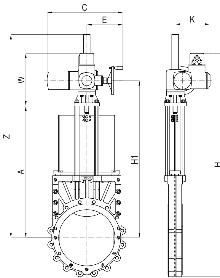
Рис. Задвижка ножевая типа TDO с электромеханическим приводом типа NE.
