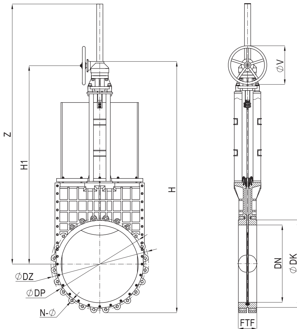
Рис. Задвижка ножевая тип TDO исполнение „wafer” / „luger”.
