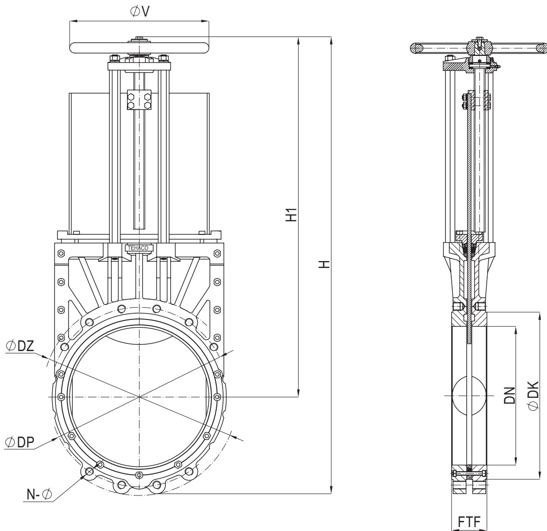
Рис. Задвижка ножевая тип TDO исполнение „wafer” - межфланцевое.
