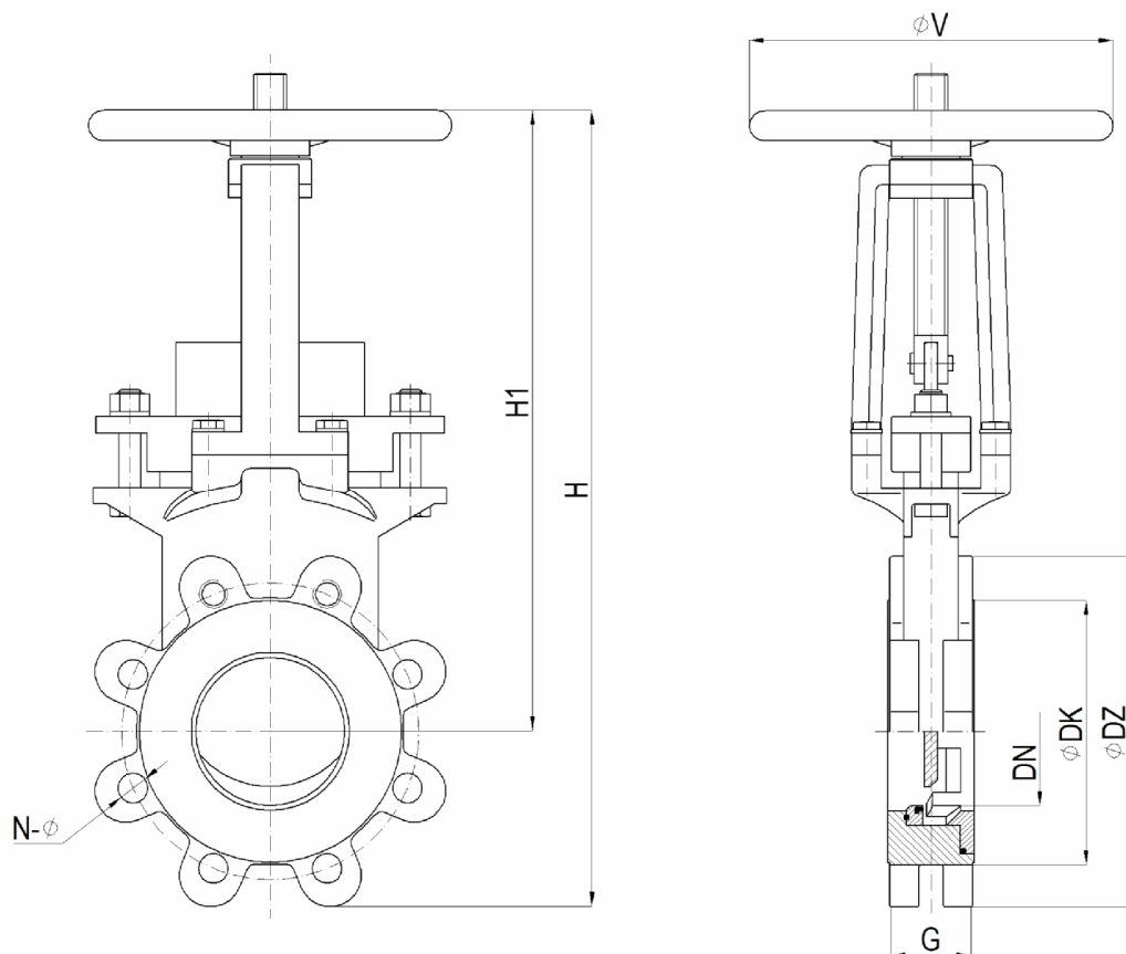
Рис. Задвижка ножевая типа TAS исполнение „luger”.
