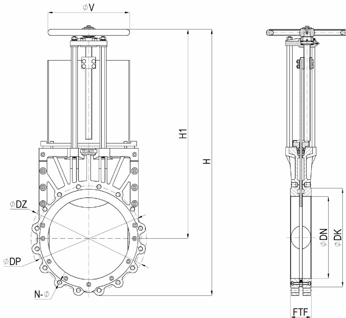
Рис. Задвижка ножевая тип TAF исполнение „luger”.
