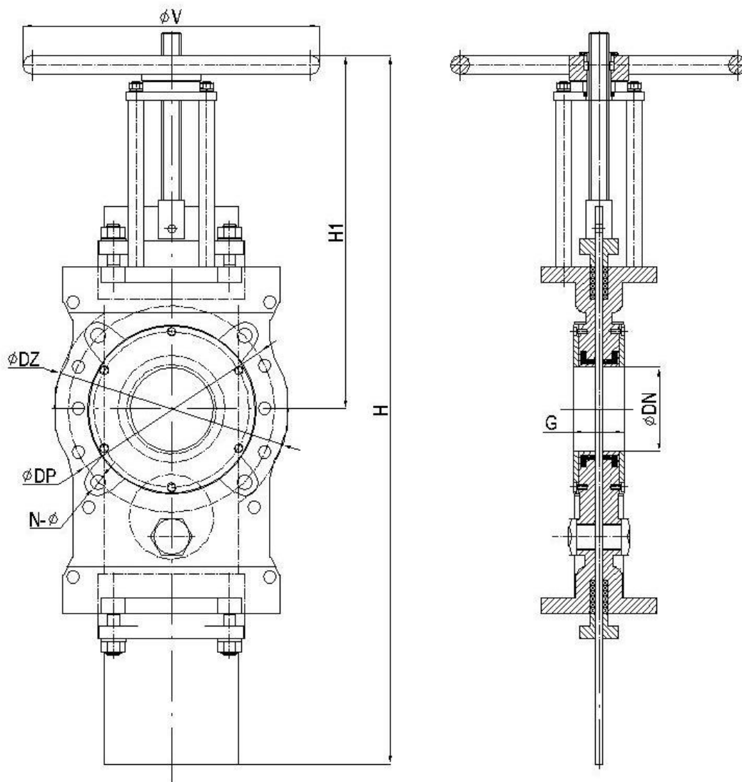
Рис. Задвижка ножевая типа HDV.
