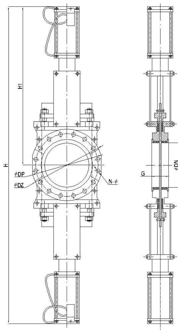
Рис. Задвижка ножевая типа DKG
