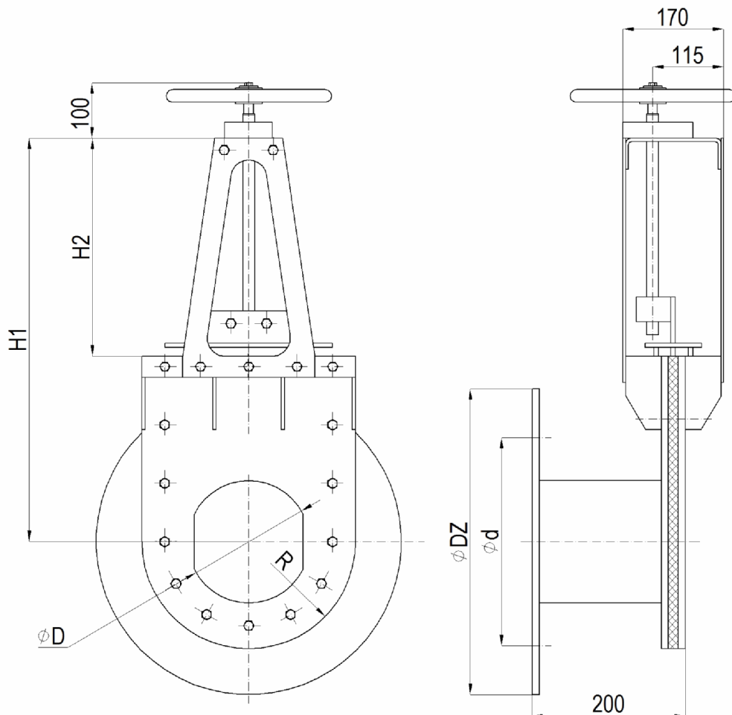
Рис. Щитовой затвор для монтажа в трубопроводе тип TZR.
