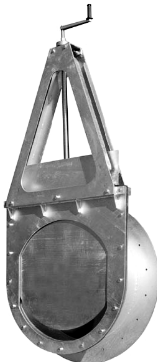
Фот. Щитовой затвор для монтажа в трубопроводе тип TZR.
