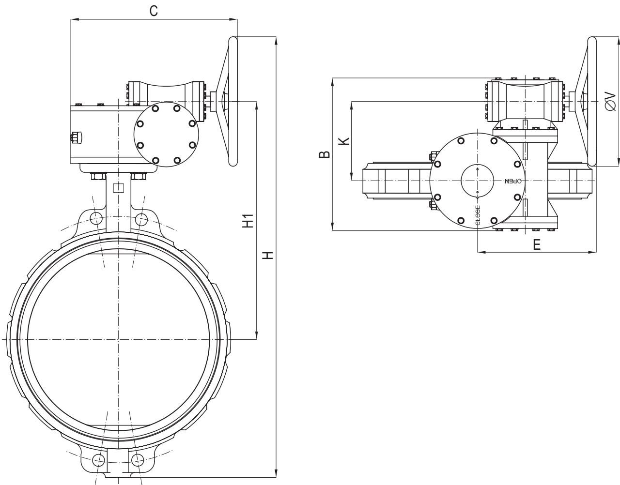
Рис. Затвор тип TCB-16 с редуктором тип GB.
