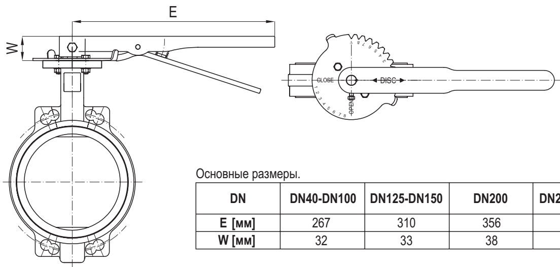
Рис. Рукоятка тип NR.
