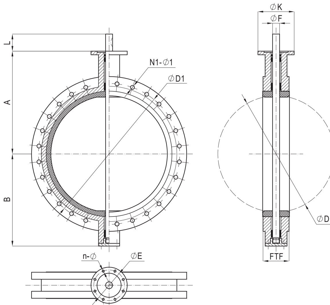
Рис. Затвор тип TCB - 16 исполнение „wafer” - межфланцевое.
