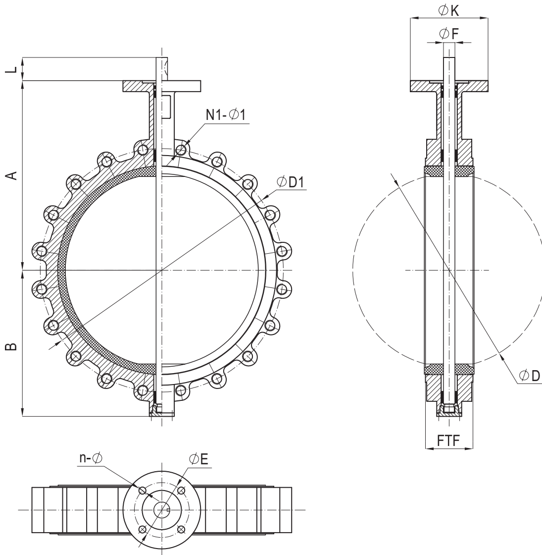
Рис. Затвор тип TCB - 16 исполнение „luger” - на конце трубопровода.
