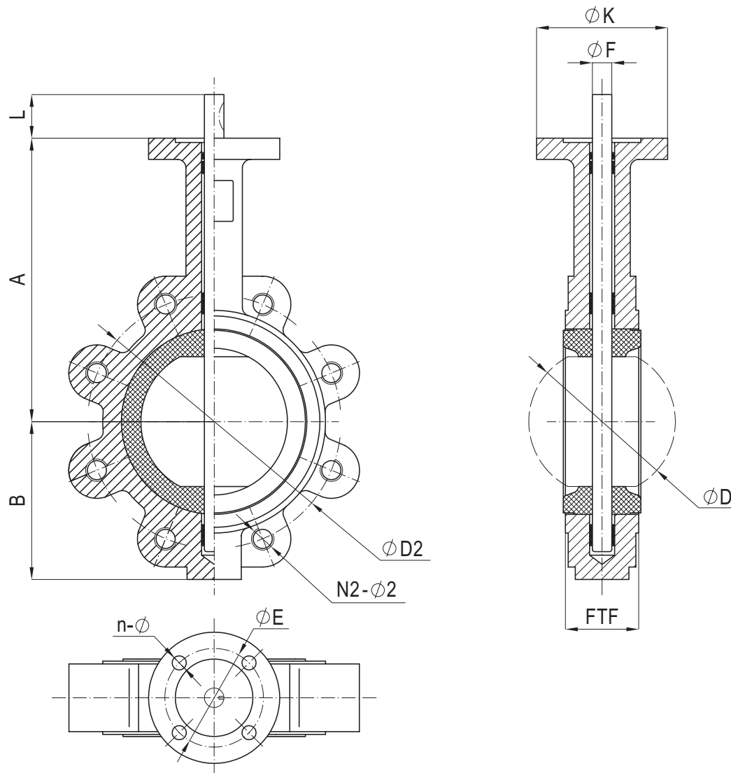
Рис. Затвор тип TCB - 16 исполнение „luger” - на конце трубопровода.
