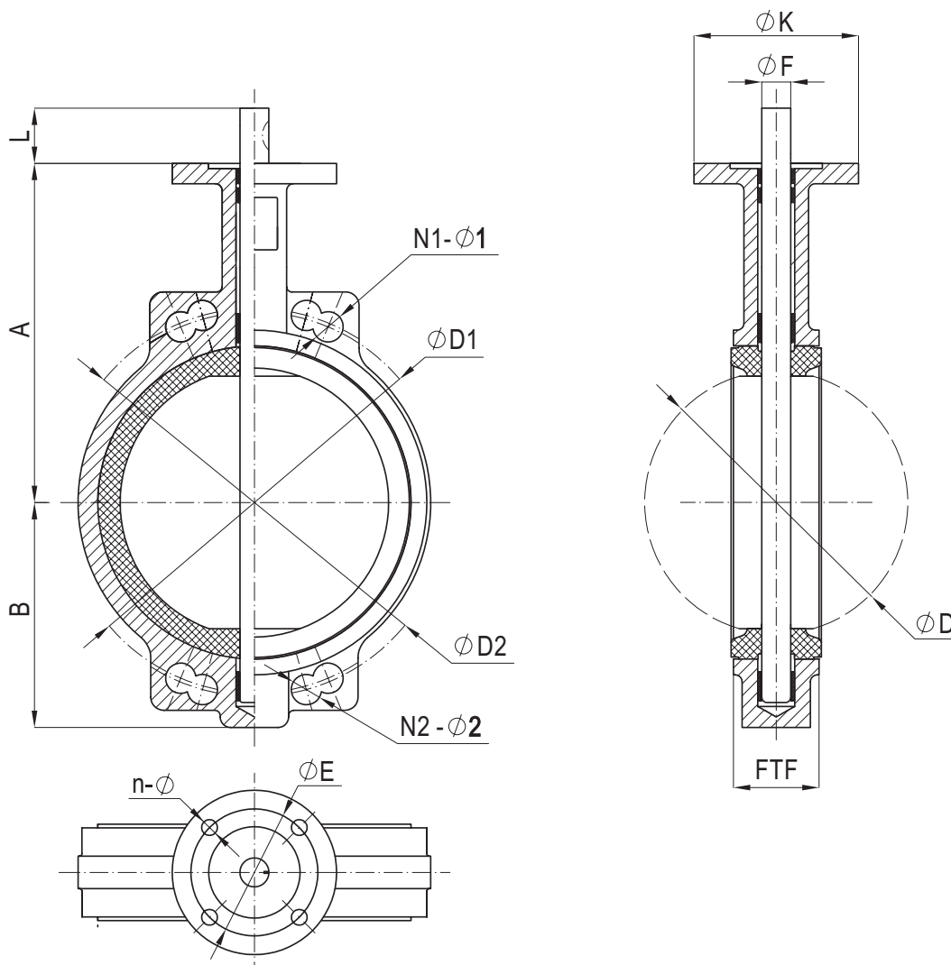
Рис. Затвор тип TCB - 16 исполнение „wafer” - межфланцевое.
