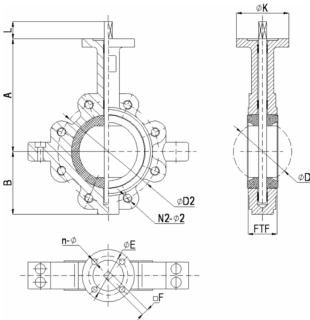
Рис. Затвор типа ТСТ, исполнение „luger”.
