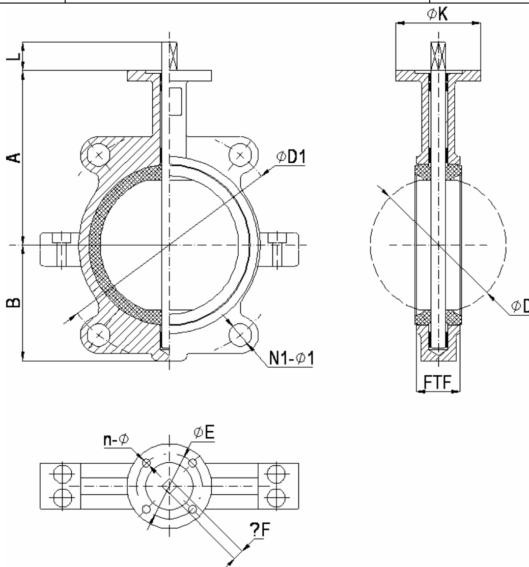
Рис. Затвор типа ТСТ, исполнение „wafer”.
