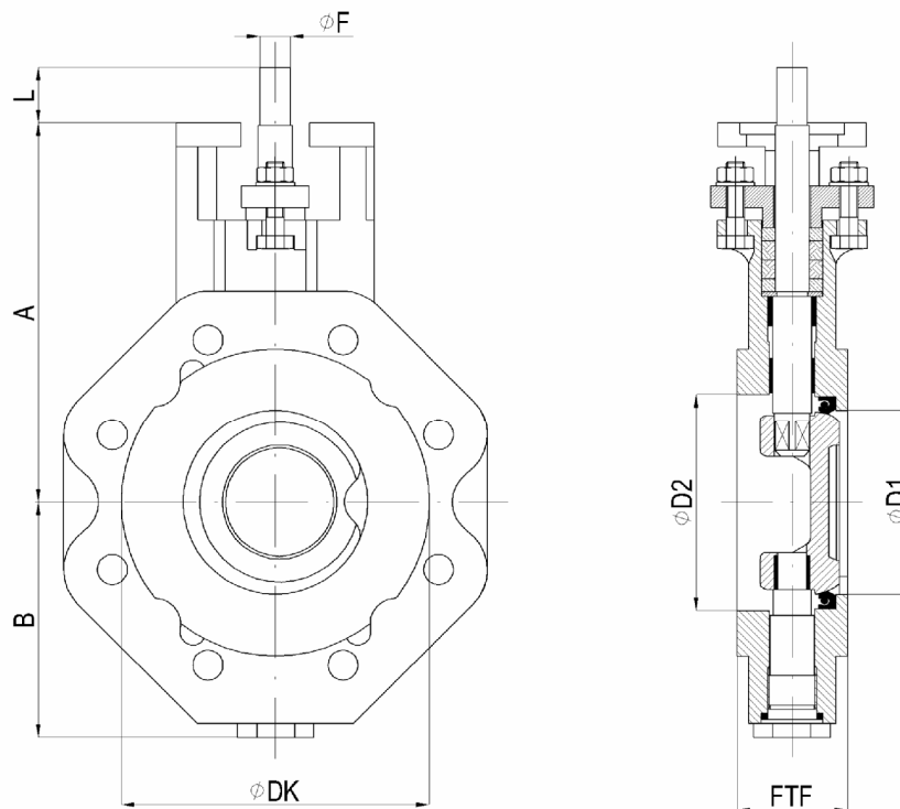
Рис. ЗАТВОР тип TCD исполнение „luger”
