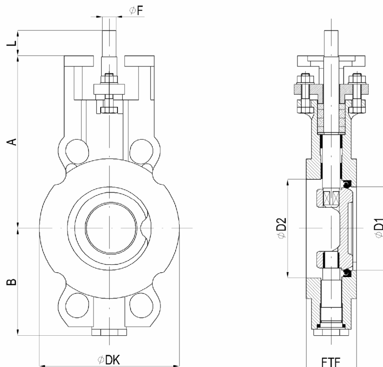
Рис. Затворы тип TCD исполнение „wafer”.
