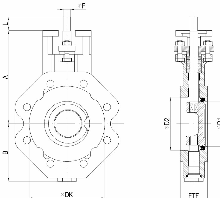
Рис. ЗАТВОР тип TCD исполнение „luger”.
