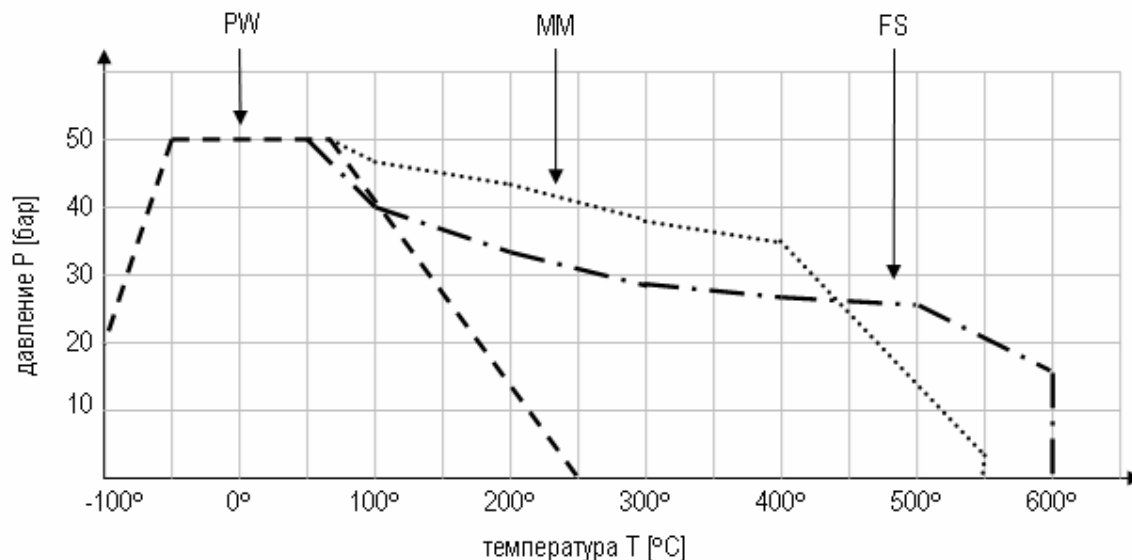
График P - T для уплотнений PW / MM / FS DN 50 – DN 100
