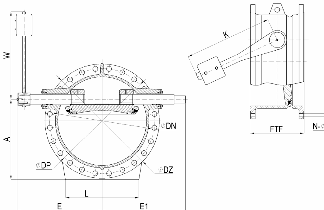
Рис. Возвратная заслона с противовесом тип KZP.
