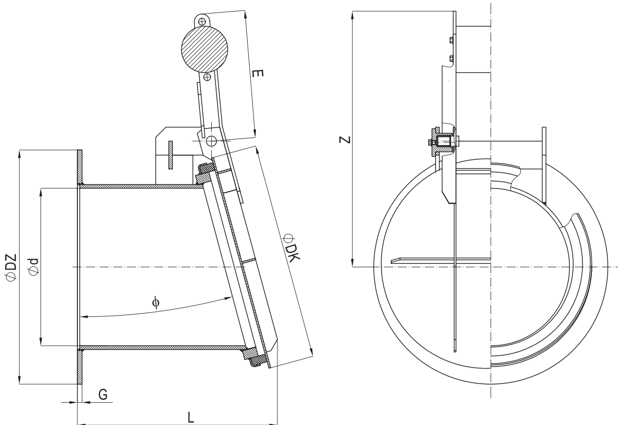
Рис. Откидной клапан тип ТКВ-BB.
