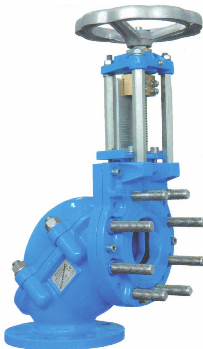
Fot. Zawór zwrotny kolanowy SZUSTER system typ TSK COMBI 02
