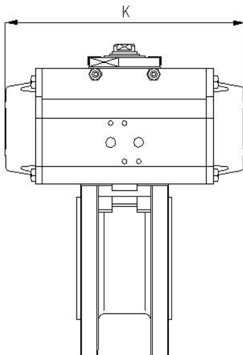
Rys. Zawór kulowy typ ZKM z napędem pneumatycznym.
