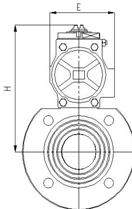
Rys. Zawór kulowy typ ZKM z napędem pneumatycznym.
