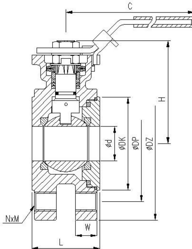
Rys. Zawór kulowy typ ZKM.
