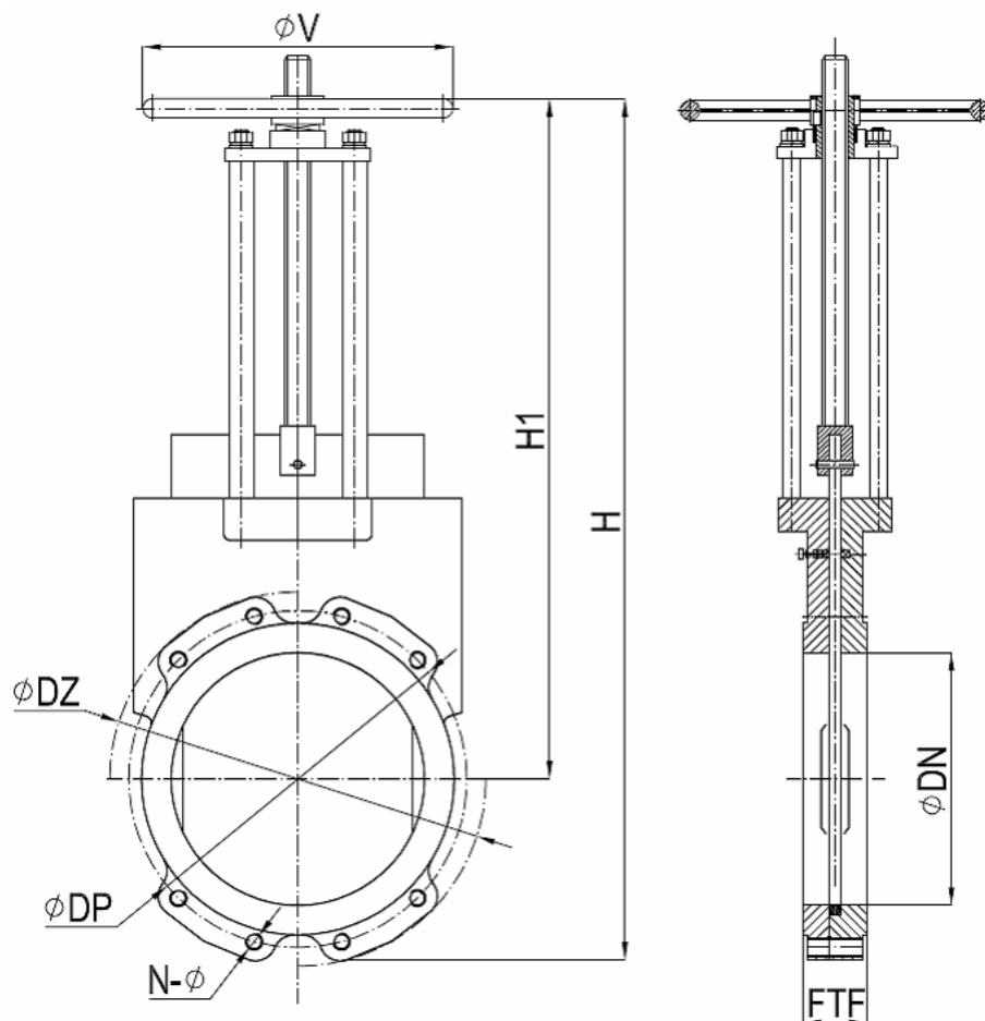
Rys. Zasuwa nożowa typ TSR wykonanie „wafer”.
