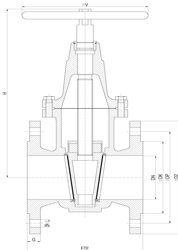
Rys. Zasuwa pierścieniowa typ TFG.
