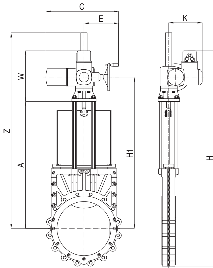
Rys. Zasuwa nożowa typ TDO z napędem elektromechanicznym typ NE.
