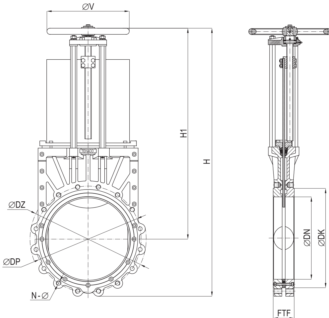
Rys. Zasuwa nożowa typ TDG-PROREM wykonanie „luger”.
