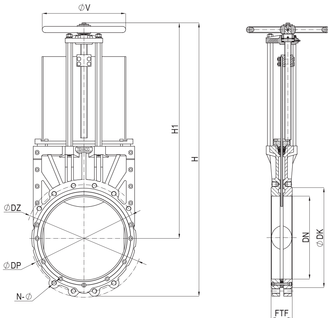
Rys. Zasuwa nożowa typ TDG-PROREM wykonanie „wafer”.
