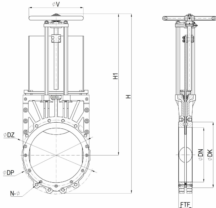
Rys. Zasuwa nożowa typ TAF wykonanie „wafer”.
