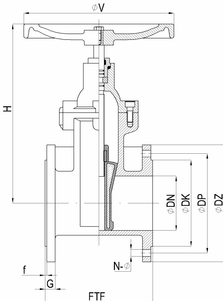
Rys. Zasuwa pierścieniowa typ RGV.
