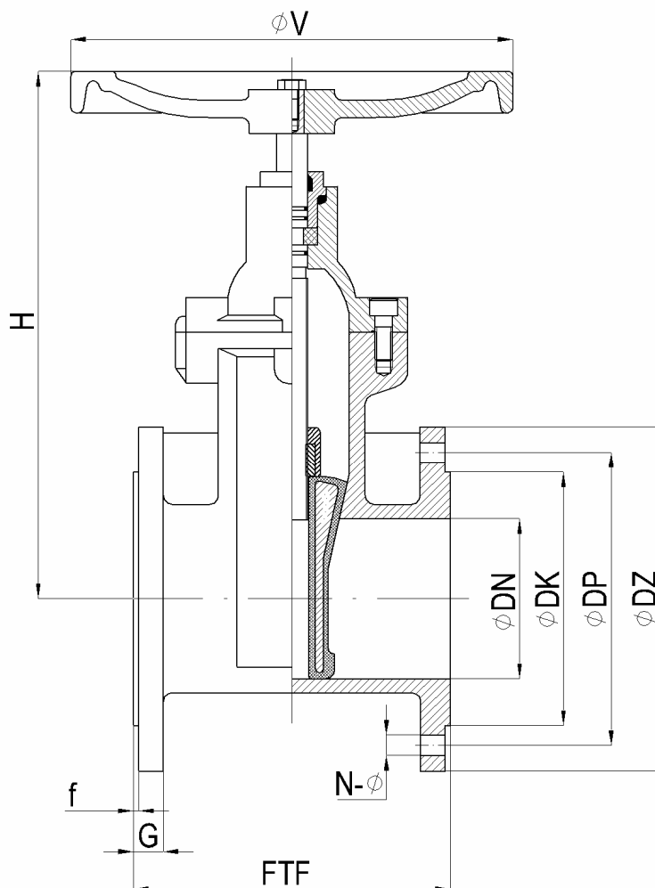
Rys. Zasuwa kołnierzowa typ RGV.
