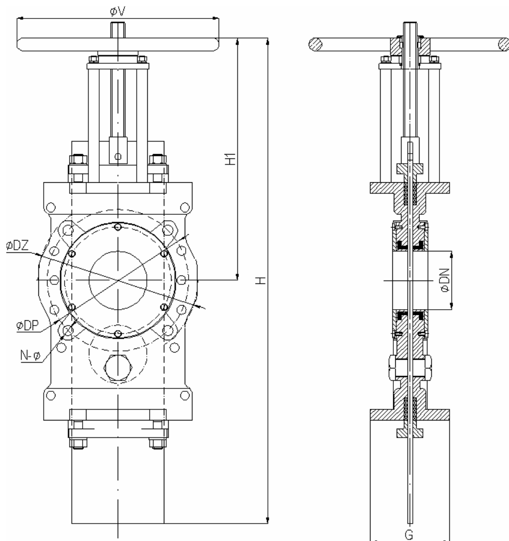
Rys. Zasuwa nożowa typ HDV.
