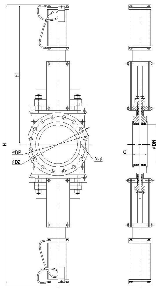
Rys. Zasuwa nożowa typ DKG.
