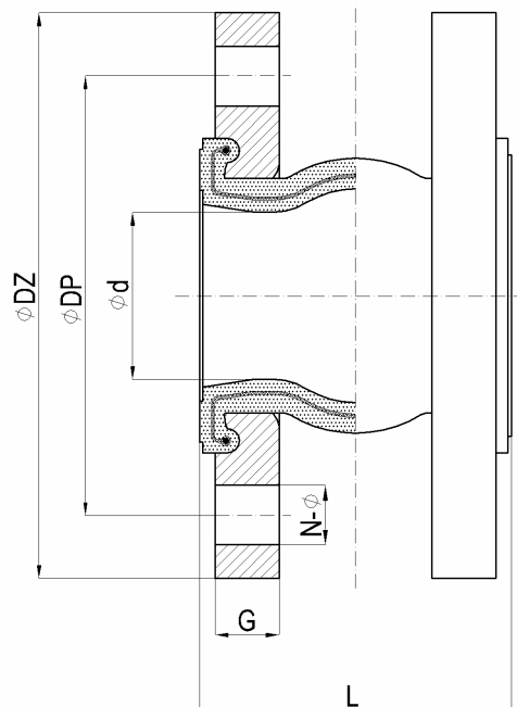
Rys. Kompensator typ TKK.
