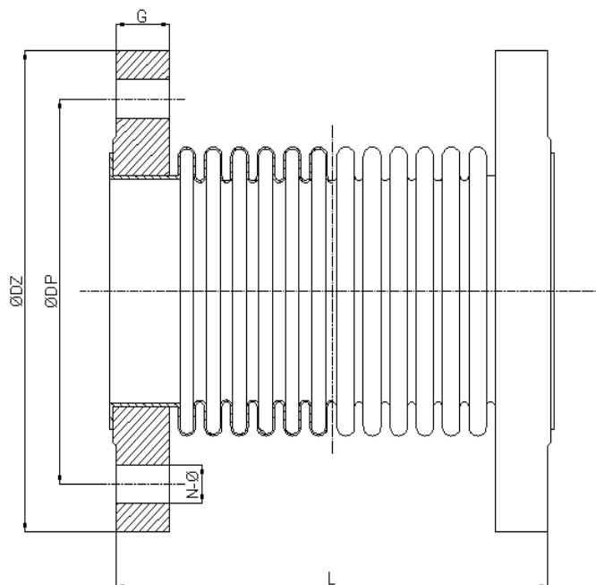
Rys. Kompensator typ SKK.
